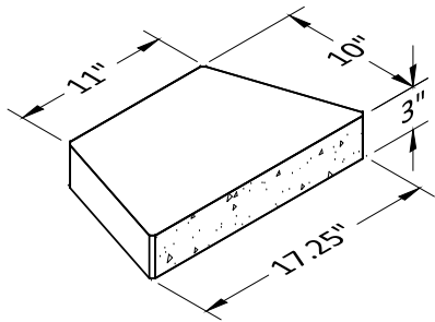
Cap Unit
