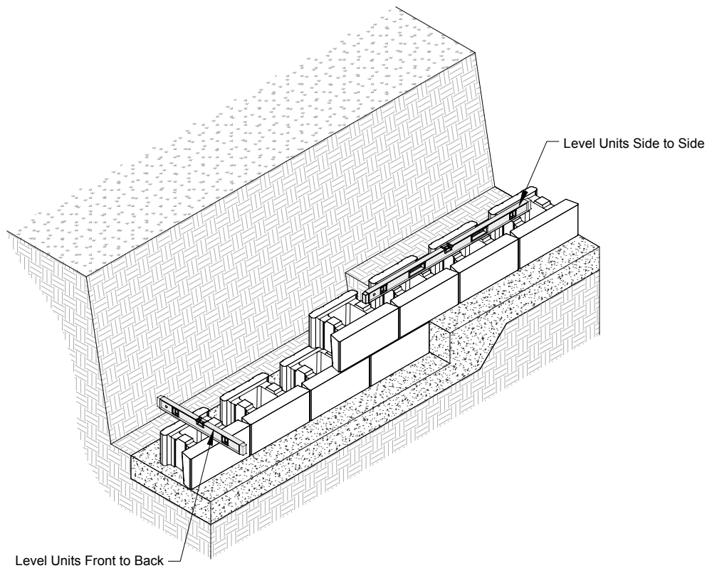
A:4 - LEVELING PAD
