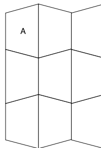
#830 4" Trapezoid Cap Pieces per layer: 9 Layers per pallet: 7
