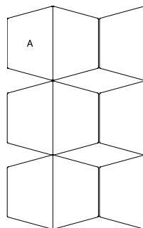
#817 3" Trapezoid Cap Pieces per layer: 9 Layers per pallet: 8
